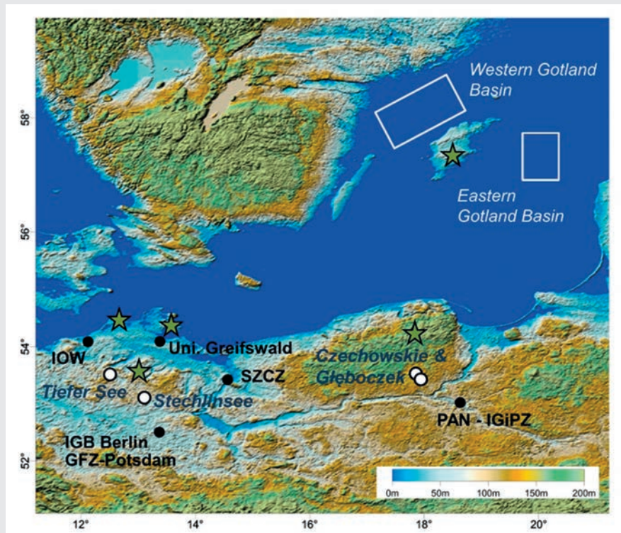
Die Untersuchungsgebiete von BaltRap: weiße Rechtecke: Beprobung von Ostsee-Sedimenten; grüne Sterne: Mooregebiete; weiße Punkte: Seen. Grafikmontage: IOW
