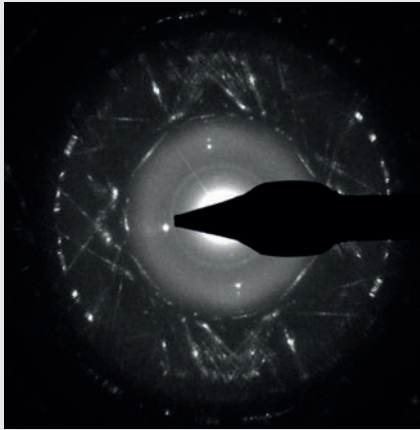
Elektronenbeugungsmuster von Vanadiumoxid nach dem Herstellungsprozess durch plasmagestützte Elektronenstrahlverdampfung.
